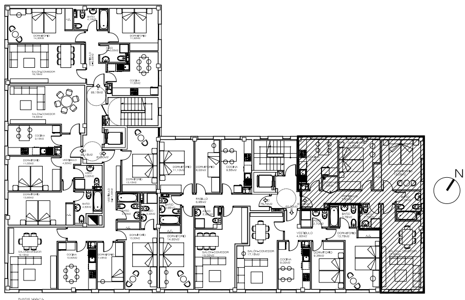
BLOQUE A. PLANTAS 1, 2, 3 Y 4. PORTAL 2 - VIVIENDA A. ESCALA 1/50 S UTIL APROXIMADA = 67,25 M 2
