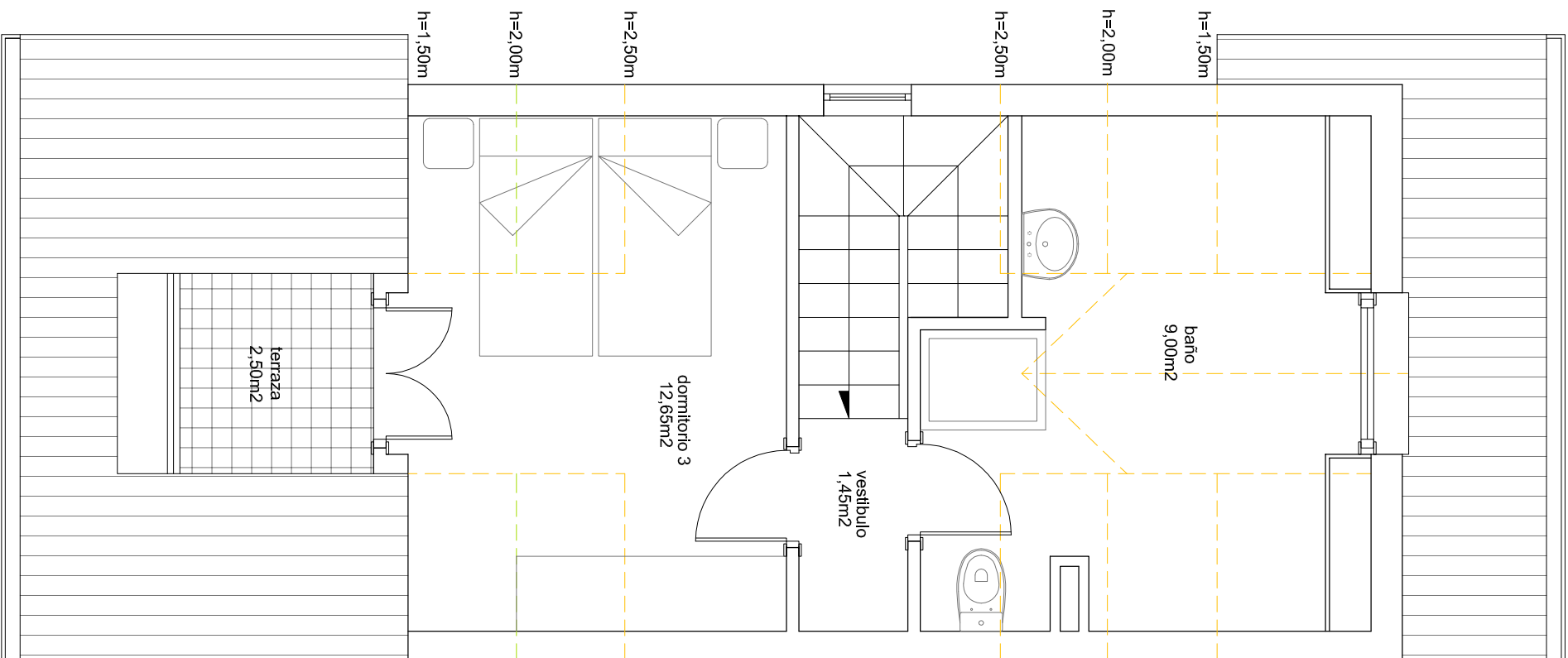
PLANTA BAJO CUBIERTA VIVIENDA 22
